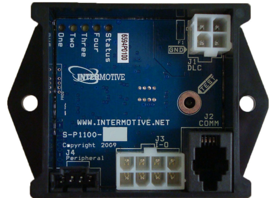
LOCK MODULE
